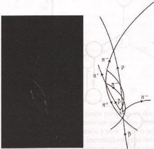
Red de reacciones que involucra protones, antiprotones, un par lambda-antilambda y varios piones.
