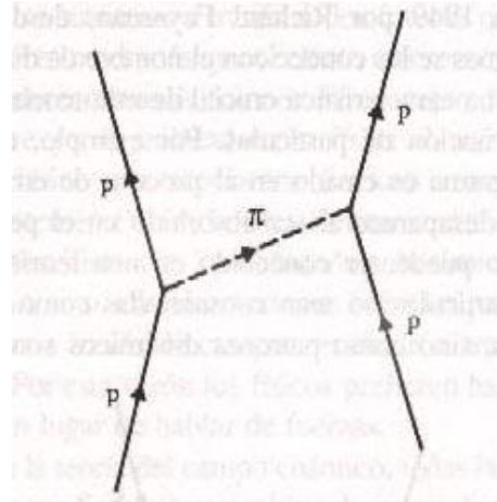
Intercambio de un pión ( \pi ) entre dos protones
