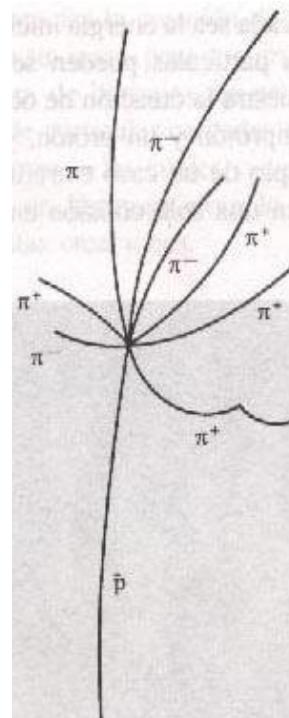
Creación de ocho piones en una colisión entre un antiprotón ( \bar{p} ) y un protón (que esperaba en la cámara de burbujas)
