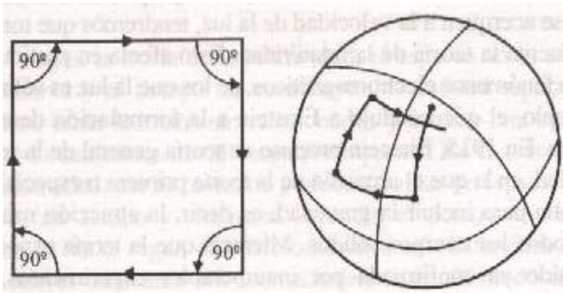
Dibujo de un cuadrado, sobre un plano y sobre una esfera
