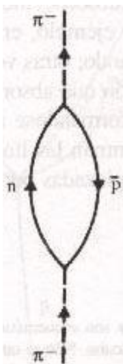
Creación de un par virtual neutrón-antiprotón
