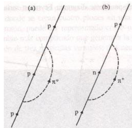
Diagramas de Feynman que muestran a un protón que emite y reabsorbe piones virtuales.
