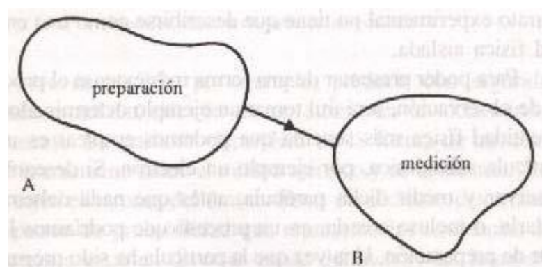
Observación de una partícula en física atómica.
