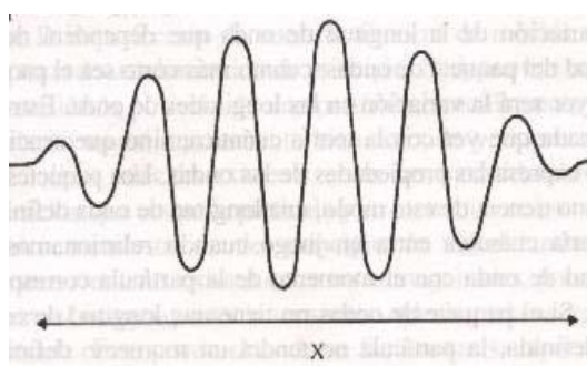
Paquete de ondas correspondiente a una partícula situada en algún lugar de la zona X
