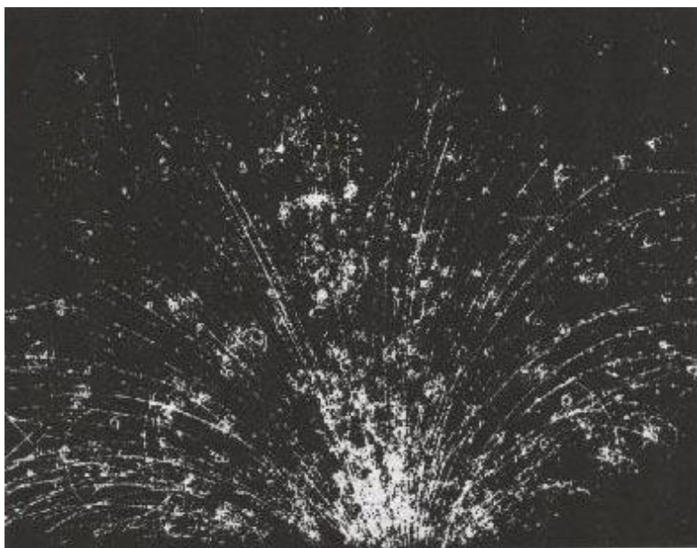
Un rayo cósmico que accidentalmente se introdujo en una cámara de burbujas provocó esta "ducha" de más de cien partículas. Los trazos horizontales corresponden a las partículas procedentes del acelerador
