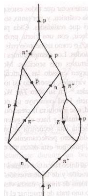
Una red de interacciones virtuales, de la obra citada de K. Ford.
