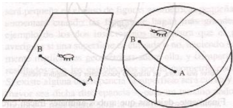
Dibujo de una "Línea Recta" sobre un plano y sobre una esfera
