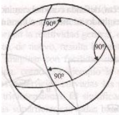
Sobre una esfera, un triángulo puede tener tres ángulos rectos
