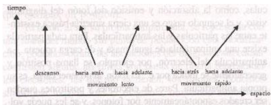
Líneas del mundo de partículas
