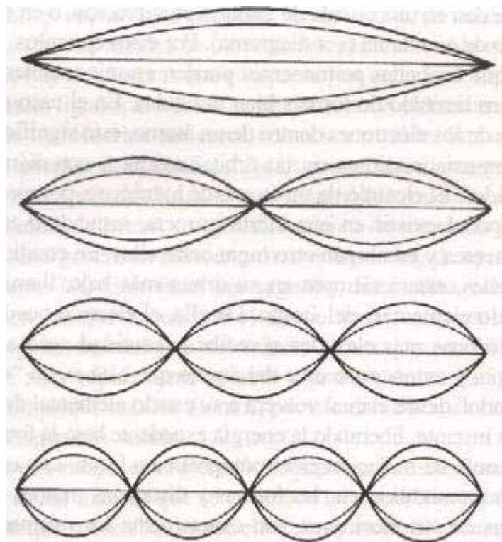
Patrones de onda permanente en la vibración de una cuerda
