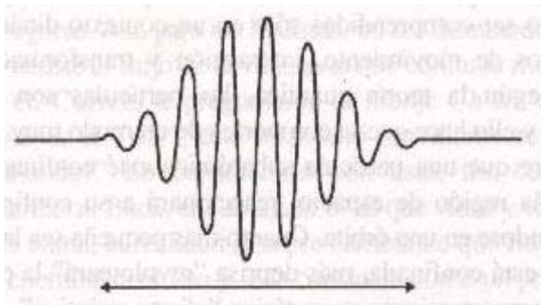
Comprimiendo el paquete de ondas dentro de una zona más pequeña
