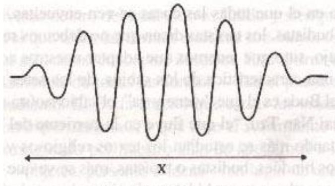
Un paquete de ondas
