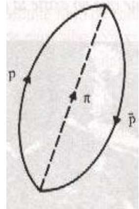
Un diagrama de vacío
